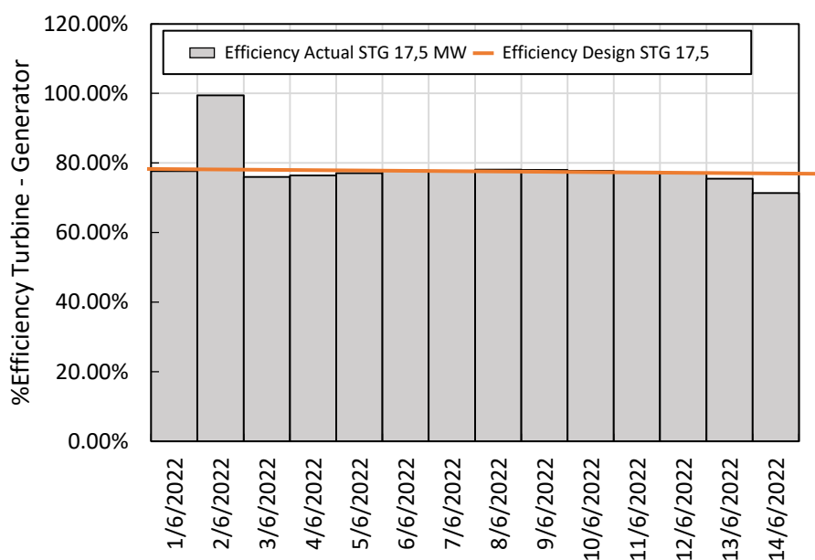
Gambar 1. Diagram waktu terhadap efisiensi steam turbine generator
