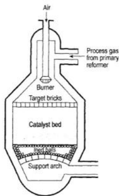
Gambar 2. Bagian Dalam Secondary Reformer [6]
