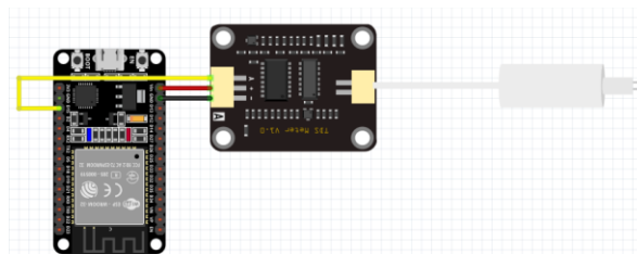
Gambar 4. Desain Elektrik Sensor TDS
