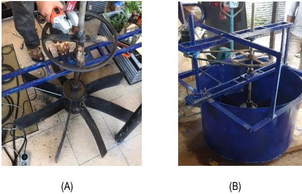
Gambar 3. 1 (A) Sudu Turbin (B) Rumah Turbin
