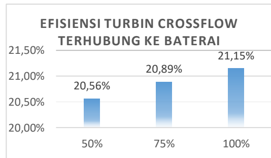
Gambar 4. 6 Efisiensi Turbin Terhubung Baterai
