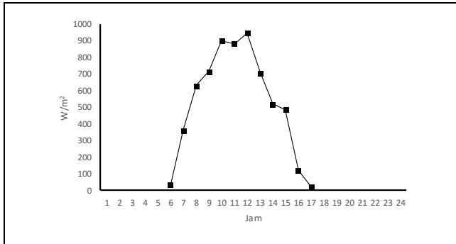
Gambar 3.2. Rata-rata intensitas radiasi matahari perjam
