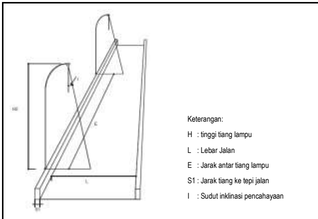
Gambar 2.1. Penempatan penerangan jalan [2]
