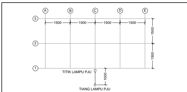
Gambar 3.3. Metode pengukuran kuat cahaya smart PJU panel surya
