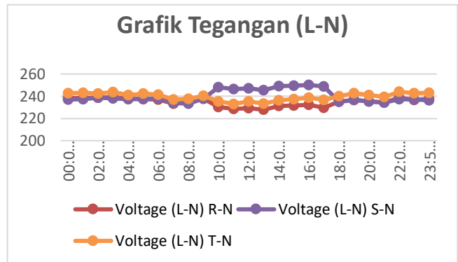
Gambar 4 Grafik Tegangan (L-N)
