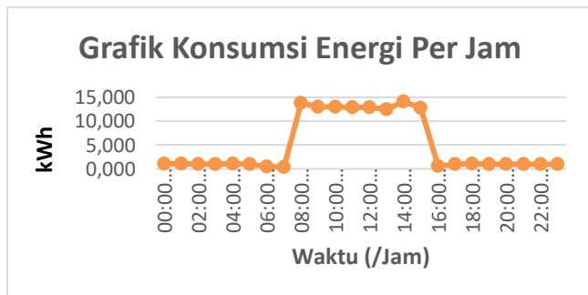
Gambar 2 Grafik Konsumsi Energi Listrik Per jam
