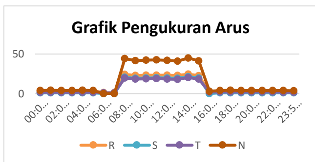
Gambar 3 Grafik Pengukuran Arus
