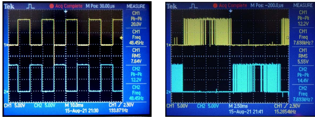
a) Luaran frekuensi dasar 50Hz
