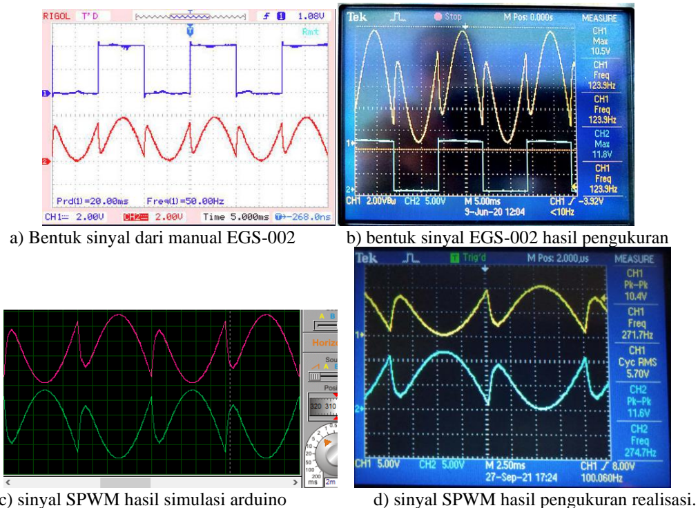
Gambar 8. Perbandingan luaran EGS-002 dengan modul SPWM berbasis arduino
