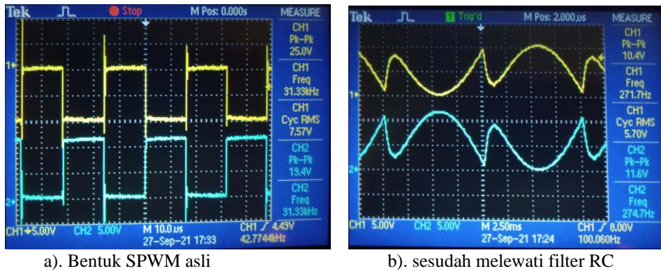
Gambar 7. Bentuk sinyal SPWM pada luaran driver
