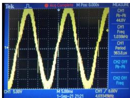
Gambar 9. Contoh output sinusoida luaran inverter sesudah melewati transformator penurun tegangan
