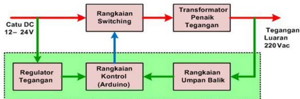
Gambar 1. Blok diagram rencana penelitian
