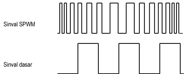
Gambar 2. Bentuk sinyal pada masing-masing pin arduino.
