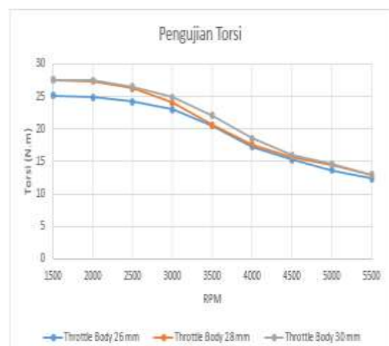
Gambar 3. Grafik Torsi
