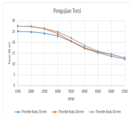
Gambar 3. Grafik Torsi
