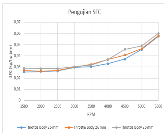
Gambar 5. Grafik SFC
