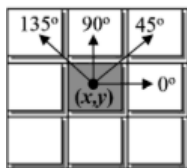
Gambar 1. Matriks GLCM dengan arah 0^\circ , 45^\circ , 90^\circ , dan 135^\circ
