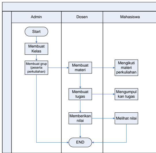
Gambar 2 Diagram Aktivitas
