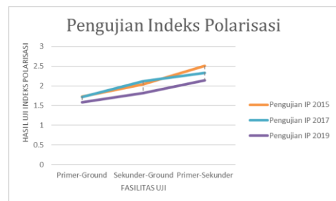
Gambar 4.4 Grafik rangkuman pengujian indeks polarisasi
