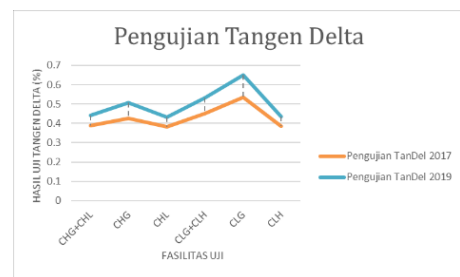
Gambar 4.5 Grafik Rangkuman Pengujian Tangen Delta Tahun 2017 dan 2019
