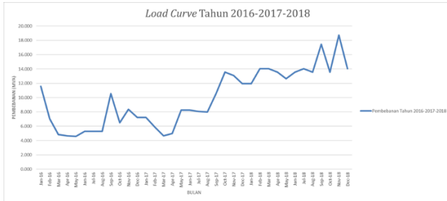
Gambar 4.1 Load Curve Transformator 1 GI Blimbing Tahun 2016-2018
