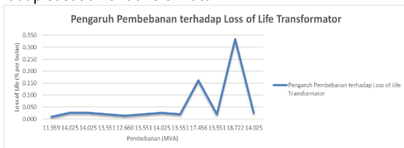
Gambar 4.2 Grafik Pengaruh Pembebanan Terhadap Loss of Life Transformator
