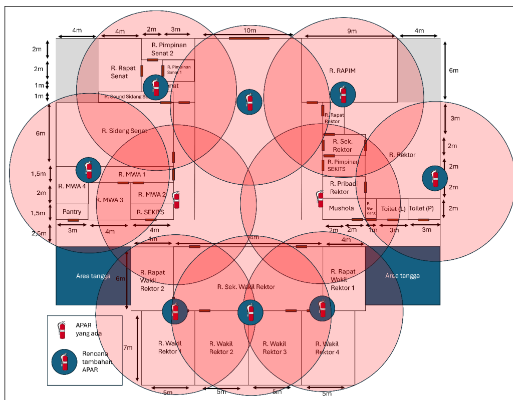
Gambar 7. Plot Penempatan APAR Kedua
