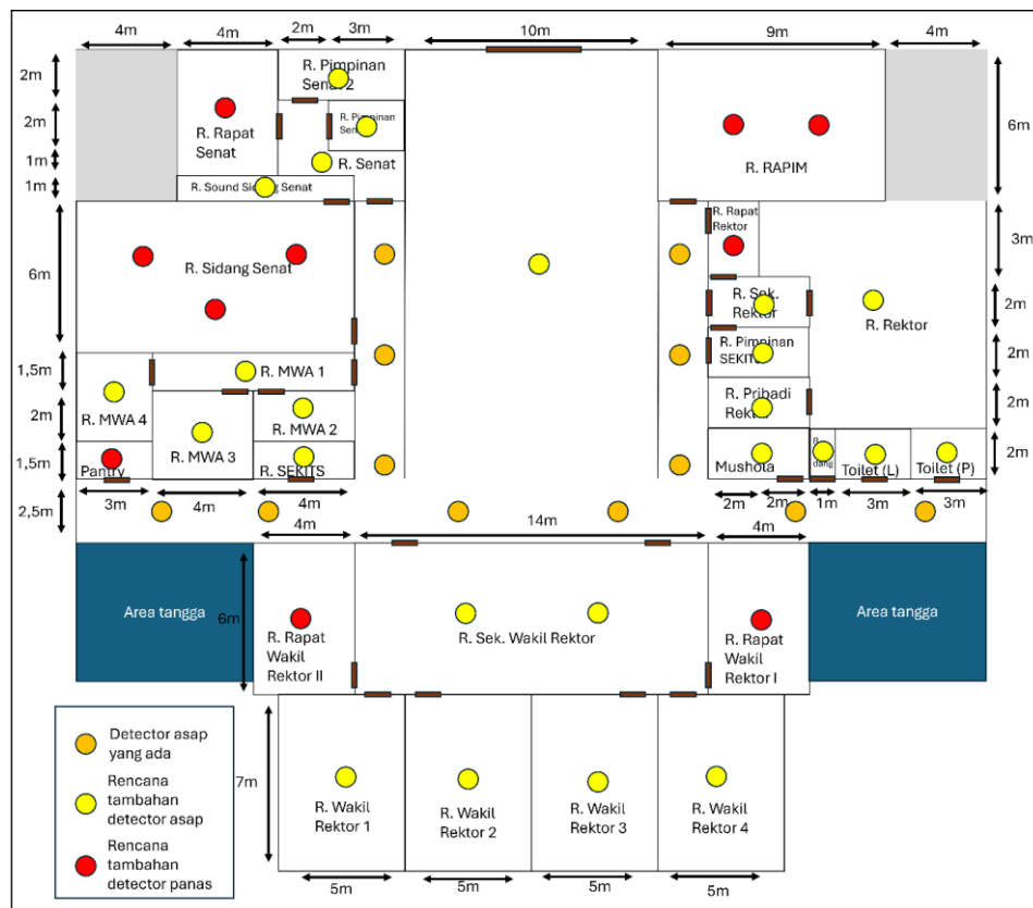
Gambar 8. Plot Penempatan Detektor Asap dan Panas.
