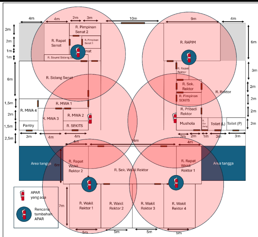
Gambar 6. Plot Penempatan APAR Pertama
