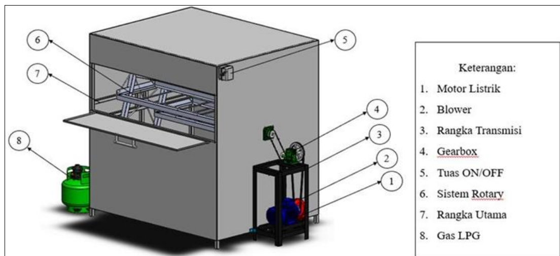
Gambar 4. Desain Mesin Oven Roti Tipe Rotari Kapasitas 120 Buah Roti
