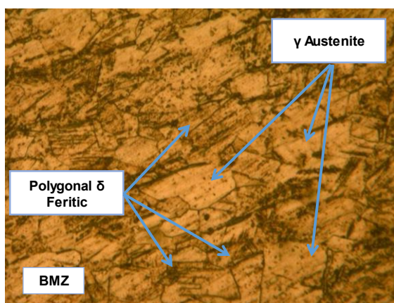
Gambar 3. Mikrostruktur Base Metal SS304
